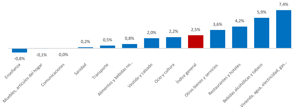
Gráfico 1. Variación interanual del IPC de Palencia por grupos. Diciembre de 2024
