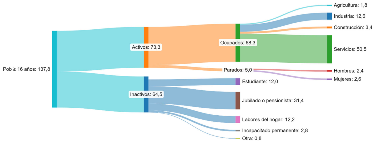
Gráfico 2. Mercado laboral de Palencia. Cuarto trimestre de 2024 (miles)
